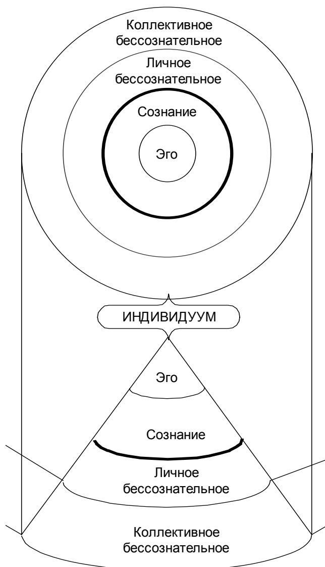
рис. 3.2. Структура психики (адаптированный материал Иоланды Якоби).
