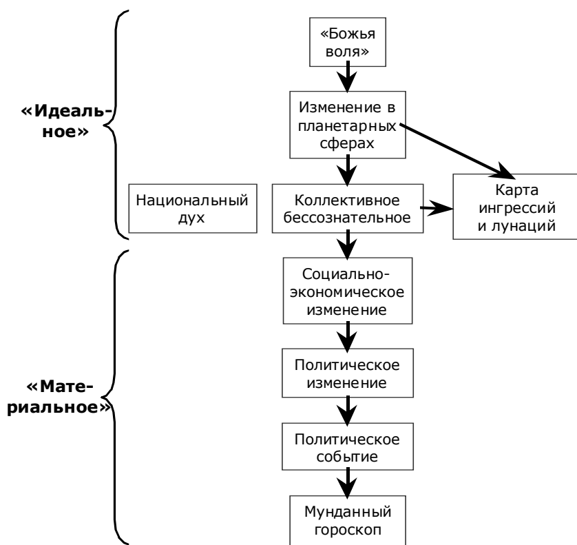
Рис. 4.2. Астрологическая модель процесса изменения в человеческом обществе
