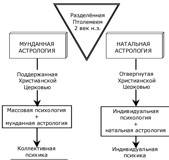
Рис. 3.4. Связь натальной и мунданной астрологии.
